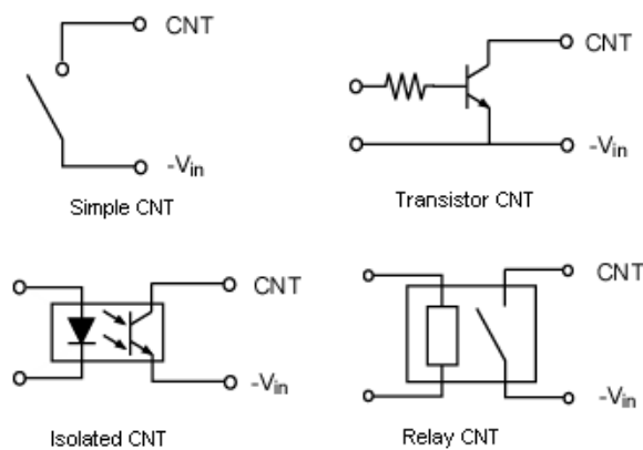
Fig. 51 CNT Circuit
