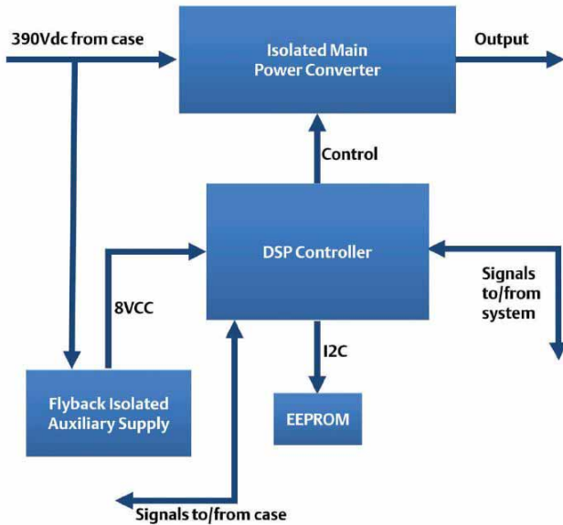
구성 가능한 전원 공급장치에서 일반적인 DSP 제어 출력 모듈의 블록 다이어그램
